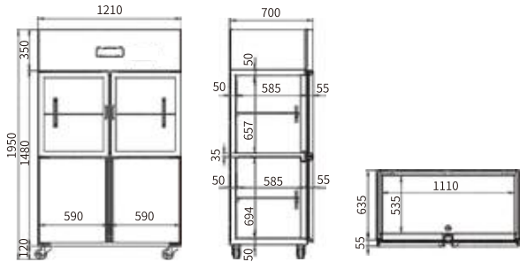
FRONT VIEW 主视图 END VIEW 侧视图 VERTICAL VIEW 俯视图
