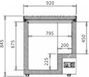
FRONT VIEW 主视图
