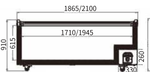
FRONT VIEW 主视图
