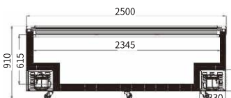
FRONT VIEW 主视图
