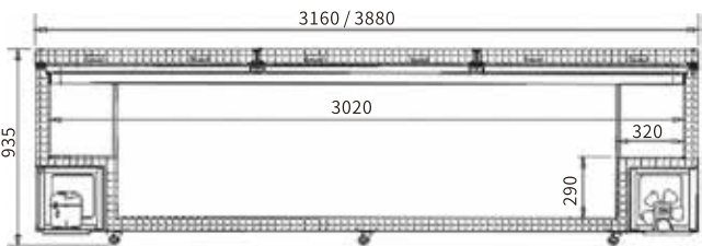
FRONT VIEW 主视图
