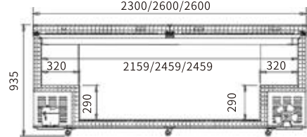
FRONT VIEW 主视图
