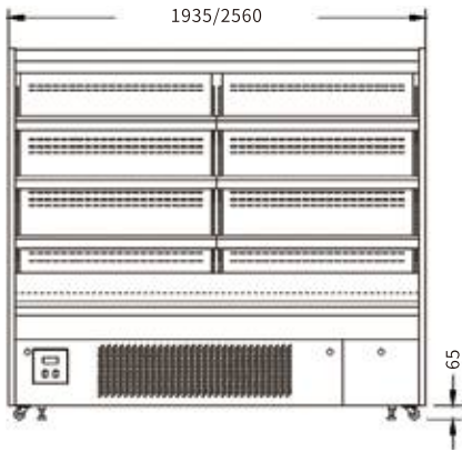
FRONT VIEW 主视图
