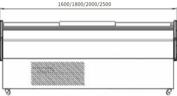
FRONT VIEW 主视图
