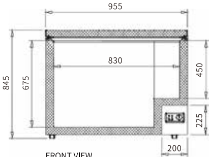
FRONT VIEW 主视图
