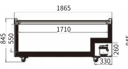
FRONT VIEW 主视图
