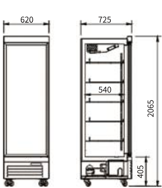
FRONT VIEW 主视图 END VIEW 侧视图
