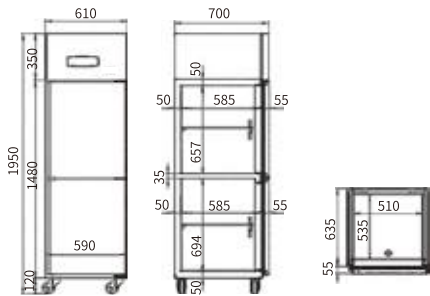
FRONT VIEW 主视图 END VIEW 侧视图 VERTICAL VIEW 俯视图
