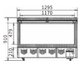
FRONT VIEW 主视图
