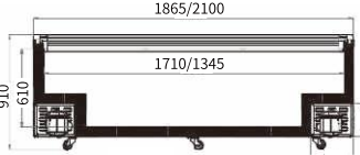
FRONT VIEW 主视图
