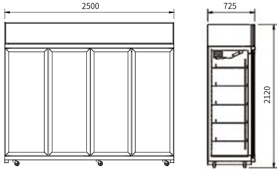
FRONT VIEW 主视图 END VIEW 侧视图
