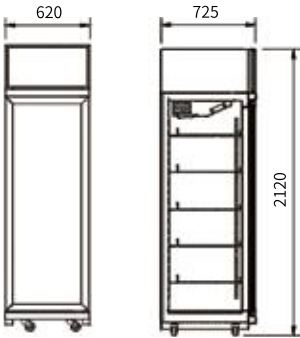
FRONT VIEW 主视图 END VIEW 侧视图
