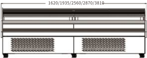
FRONT VIEW 主视图
