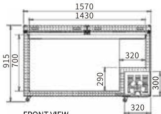
FRONT VIEW 主视图
