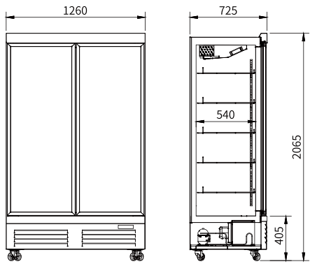
FRONT VIEW 主视图 END VIEW 侧视图
