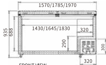
FRONT VIEW 主视图
