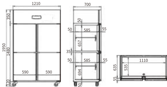
FRONT VIEW 主视图 END VIEW 侧视图 VERTICAL VIEW 俯视图
