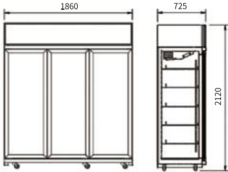
FRONT VIEW 主视图 END VIEW 侧视图
