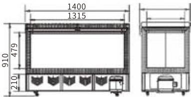
FRONT VIEW 主视图
