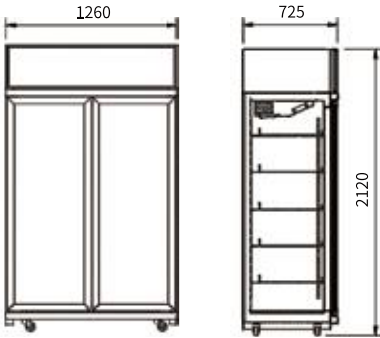
FRONT VIEW 主视图 END VIEW 侧视图
