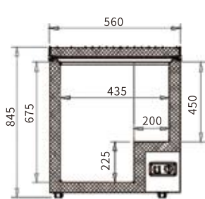
FRONT VIEW 主视图
